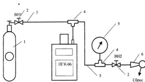
Схема Б.2 газовая для определения погрешности измерения давления (Для газоанализаторов с индексом P2).
